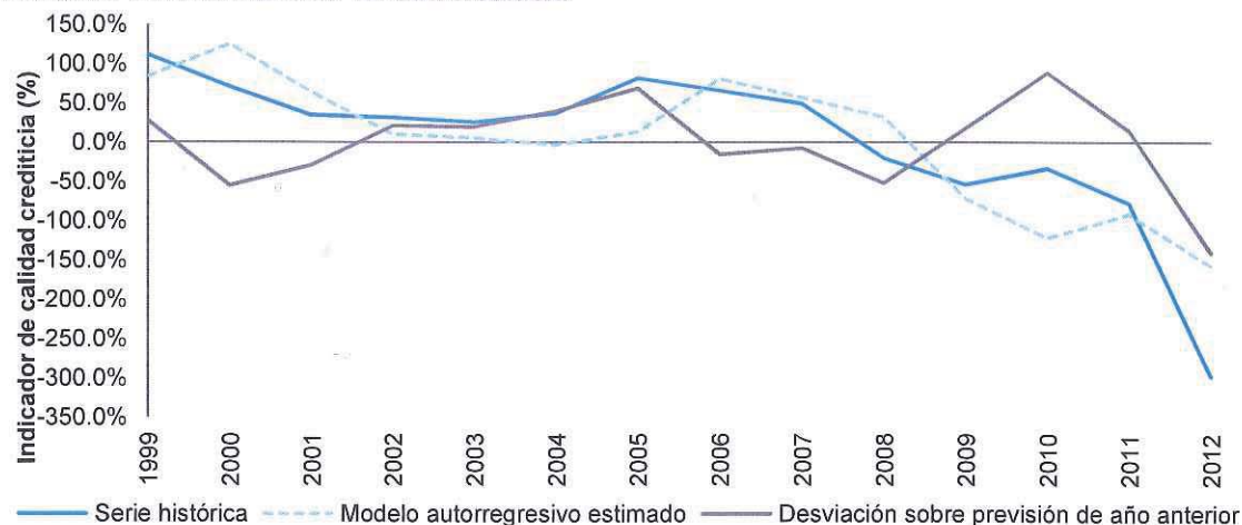
Indicador transformado de calidad crediticia
